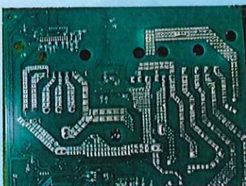
強化基板大電流處走向 基板銅箔線雙面加錫，增加 基板穩定性及壽命。
