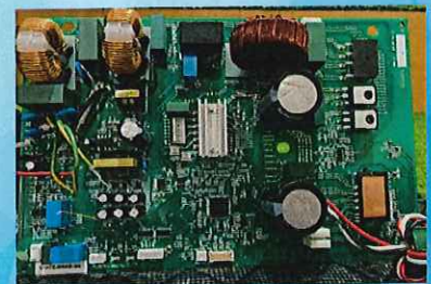
首創DC直流高壓電保護 當室外機停止運轉時，基板 會將DC直流高壓電放電，可 防止維修人員觸及高壓電、 增加變頻電子基板壽命及節 能效果。
