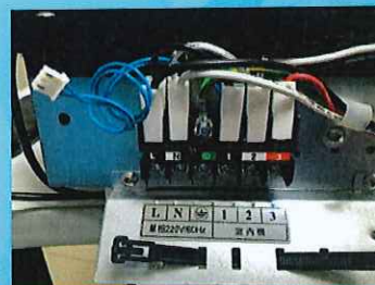
AC電源端子台過熱保護 溫度保險絲自動斷開溫度為 102°C，防止安裝配線不當及配 線老舊所產生的高溫的安全防護。
